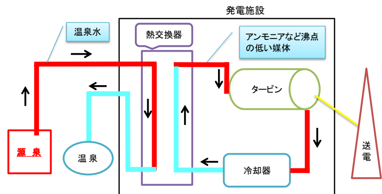
（図表4）温泉バイナリー発電のイメージ
